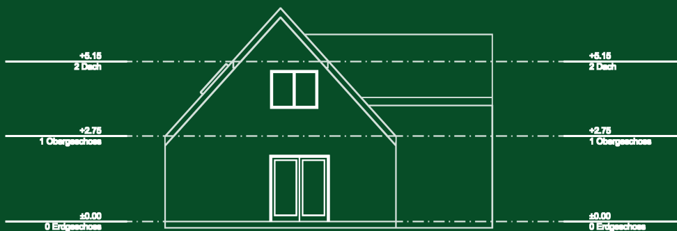
Westansicht 1:100
