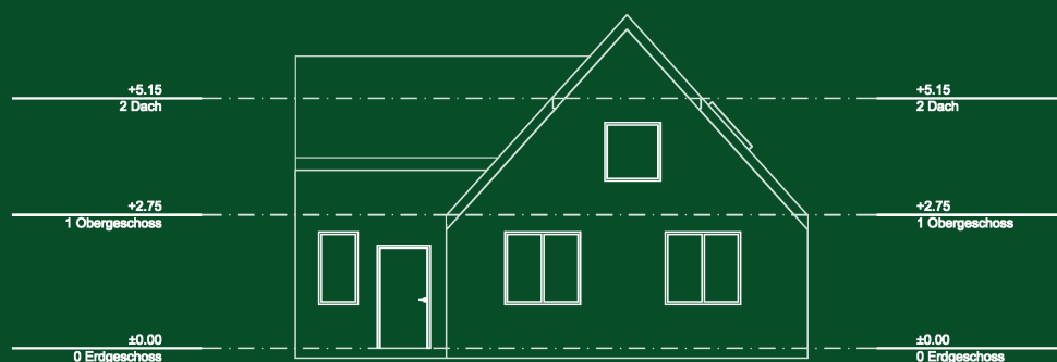
Ostansicht 1:100
