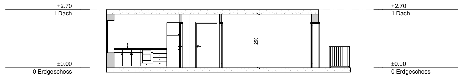
Schnitt 01 1:100
