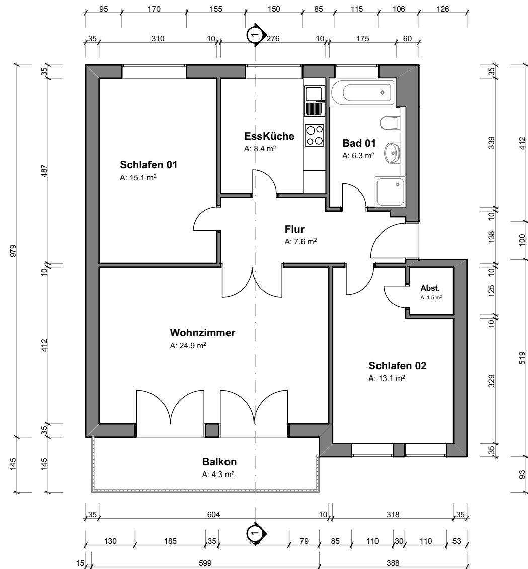
Wohnung 1:100
