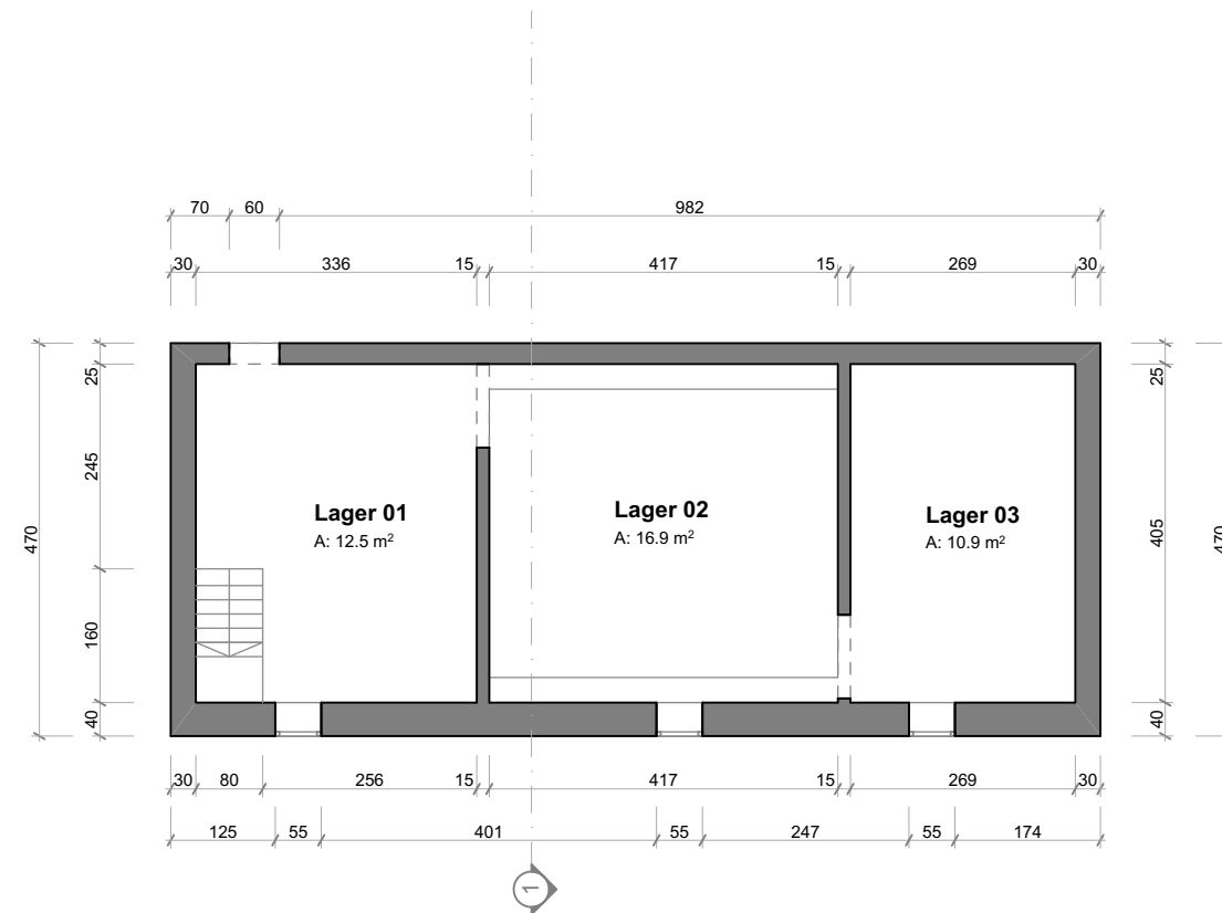
Kellergeschoss 1:100
