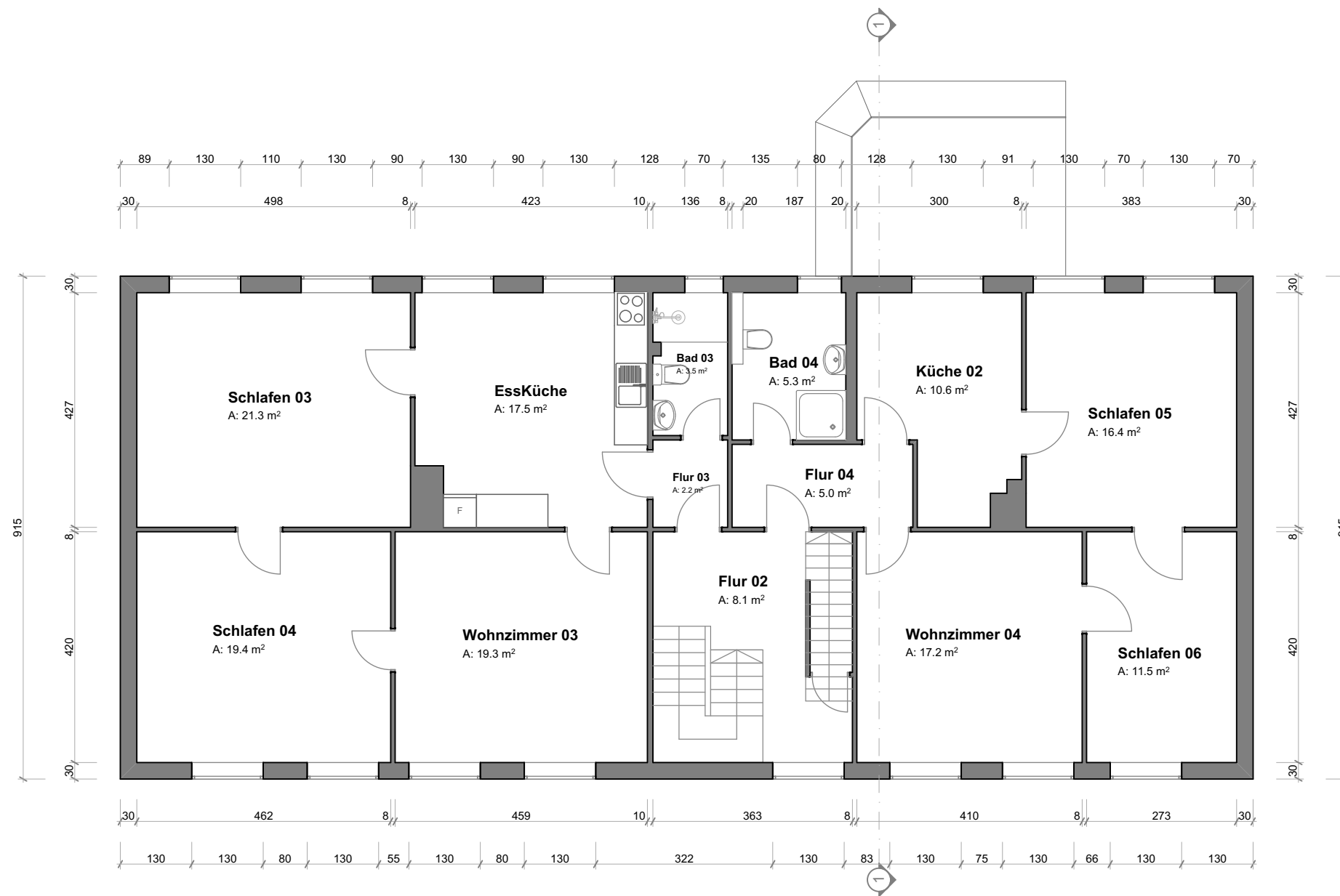
Obergeschoss 1:100
